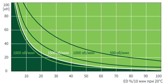
Передаточное отношение „N“ (9:1)
