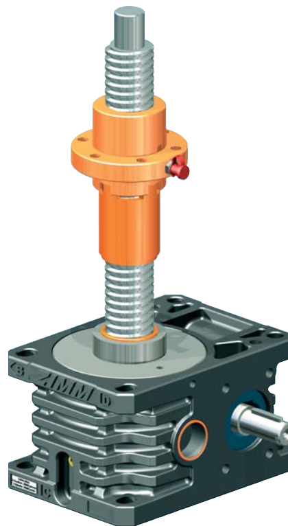
Домкрат с предохранительной гайкой SIFA
