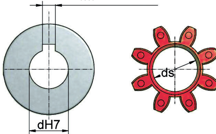
Шпоночный паз по DIN 6885
